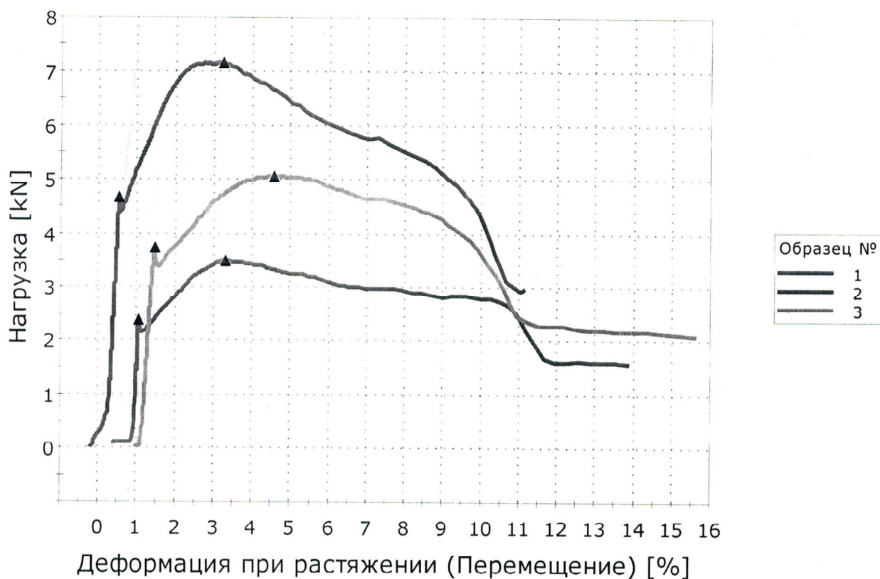
Рисунок 2 Диаграммы испытаний «нагрузка-перемещение» по определению сдвиговой нагрузки при растяжении образцов изделий «Зажим» установленный на деталь «Тяга» при -60^{\circ}\text{C}
