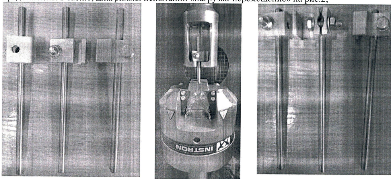
Рисунок 1 Внешний вид образцов изделий «Зажим» установленный на деталь «Тяга» при 20 \pm 5 °C
