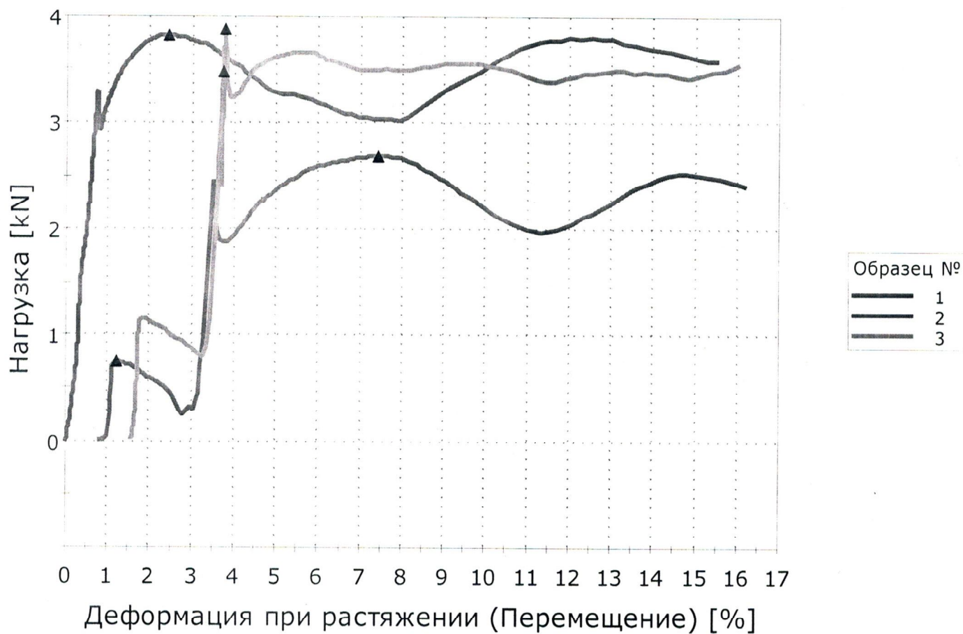
Рисунок 2 Диаграммы испытаний «нагрузка-перемещение» по определению сдвиговой нагрузки при растяжении образцов изделий «Зажим» установленный на деталь «Тяга» при 20 \pm 5 °C
