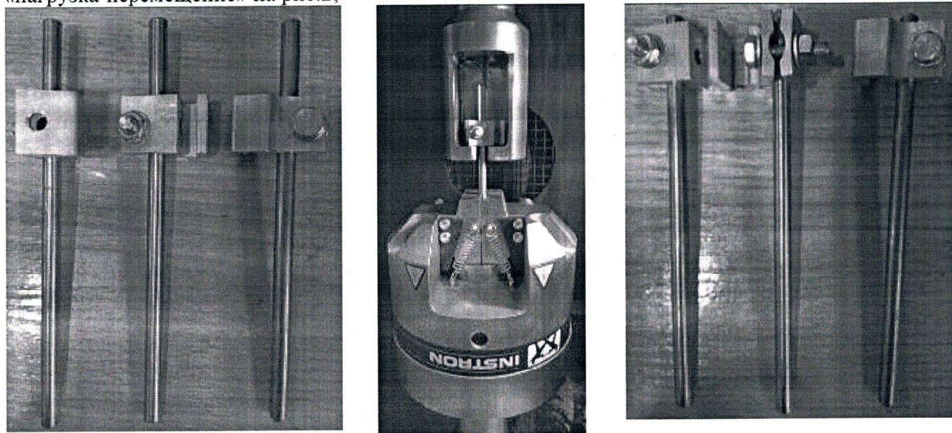
Рисунок 1 Внешний вид образцов изделий «Зажим» установленный на деталь «Тяга» после 100 циклов воздействия температуры в диапазоне -60^{\circ}\text{C} +60^{\circ}\text{C}
