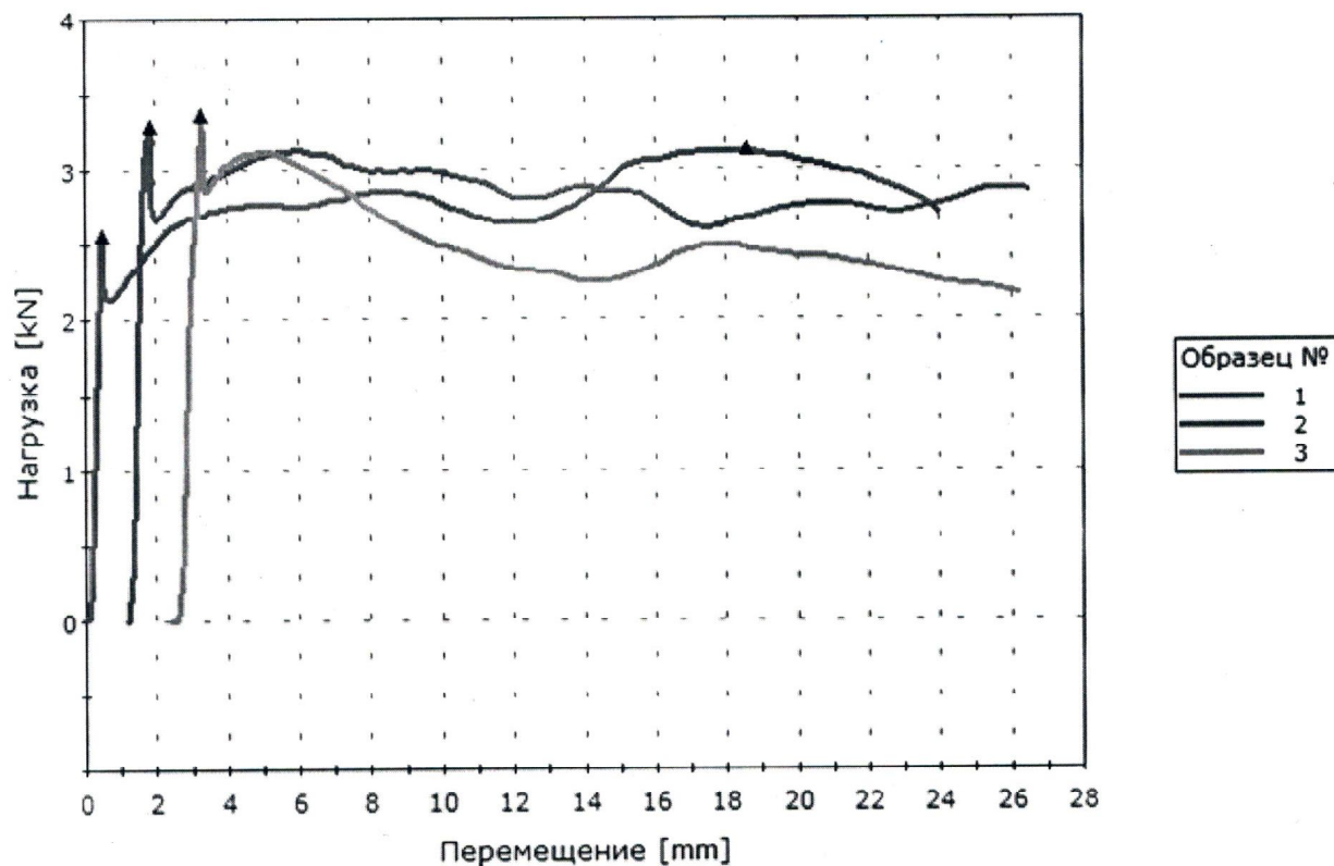
Рисунок 2 Диаграммы испытаний «нагрузка-перемещение» на определение сдвиговой нагрузки при растяжении образцов изделий "Зажим" установленный на деталь "Тяга" после 100 циклов воздействия температуры в диапазоне -60^{\circ}\text{C} +60^{\circ}\text{C}
