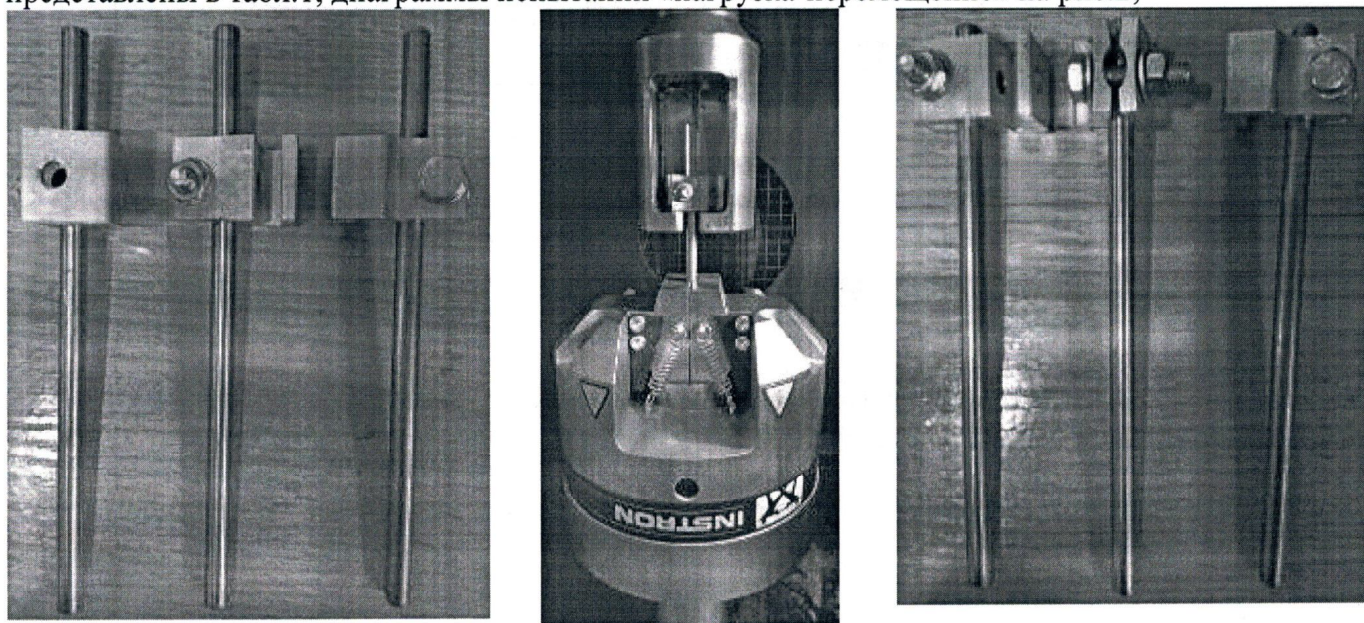
Рисунок 1 Внешний вид образцов изделий «Зажим» установленный на деталь «Тяга» при 60°С
