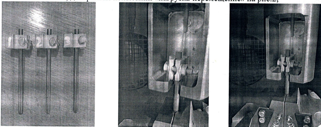
Рисунок 1 Внешний вид образцов изделий «Зажим» установленный на деталь «Тяга» при -60^{\circ}\text{C}
